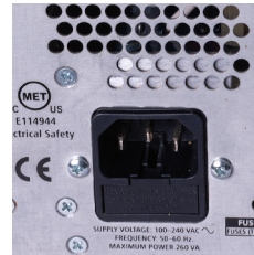
Module d'entrée d'alimentation porte-fusibles
